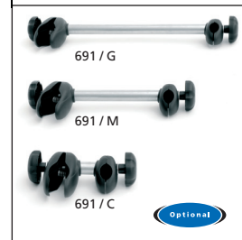
art. 691 Braccetti per fissaggio bici disponibili in 3 lunghezze versione economica Bike grab arms available separately, 3 lengths available economic version
